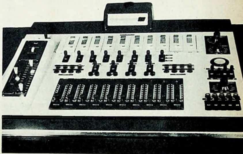
Afb. 3. Close-up van het in de foto van de regietafel in opgeklapte stand getoonde schakelpaneel.
