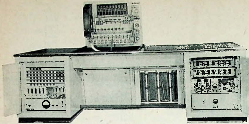
Afb. 2. De regietafel van de grote studiozaal van Radio Luxemburg.
