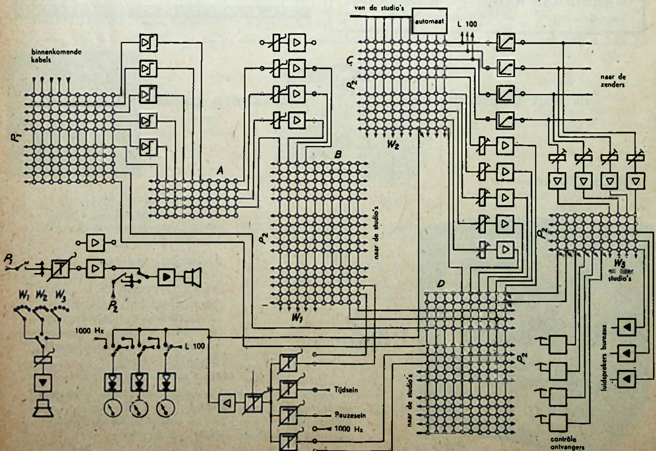
Afb. 5 SCHEMA HOOFDVERDEELRUIMTE
